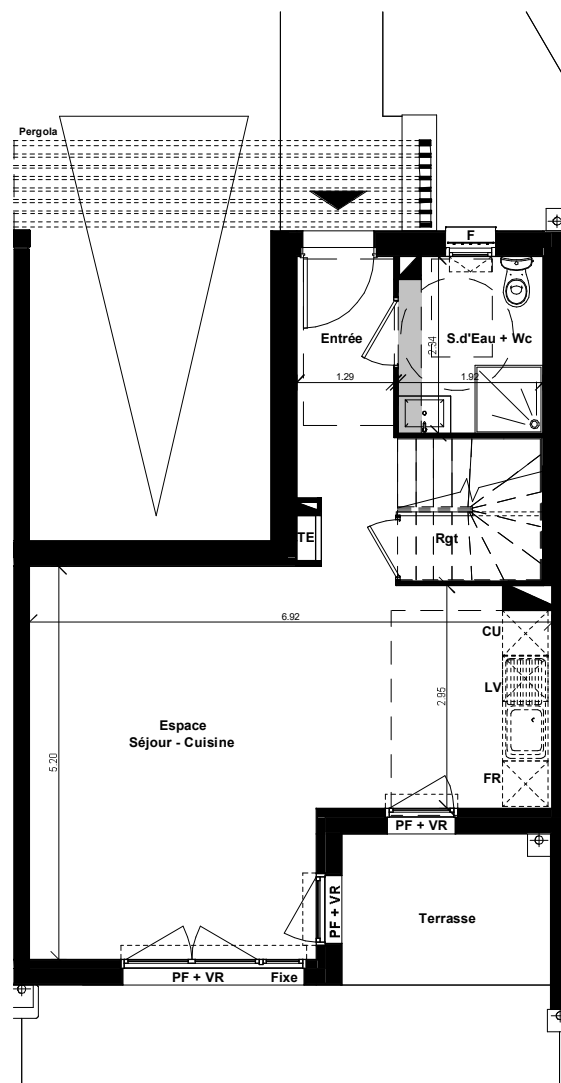
PLAN RDC
